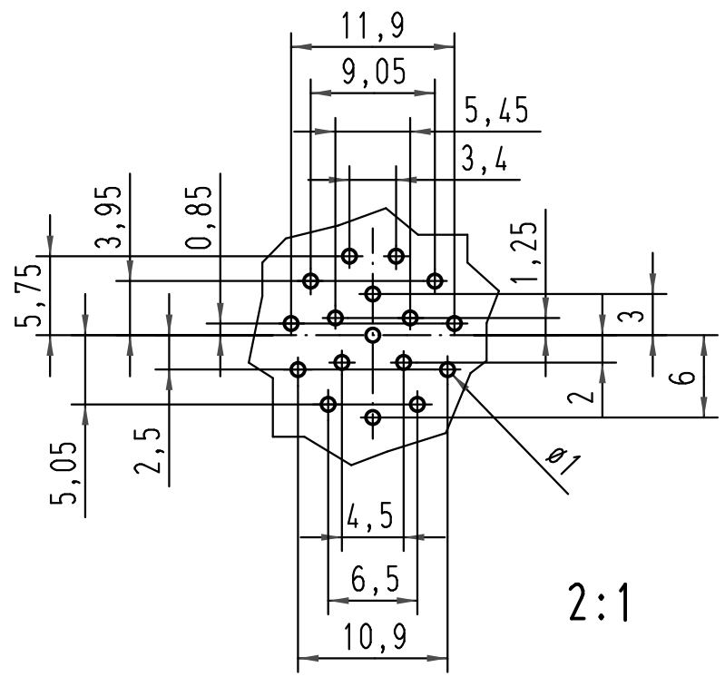
Lochbild/pinhole pattern
